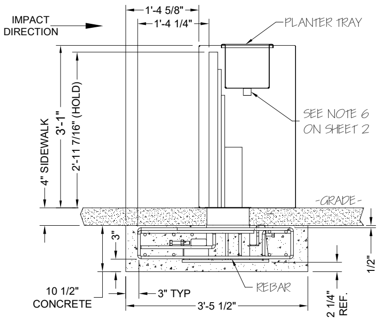
3 SIDE VIEW PL-40-003-1 Scale: None
