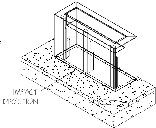
4 ISOMETRIC VIEW PL-40-003-1 Scale: None
